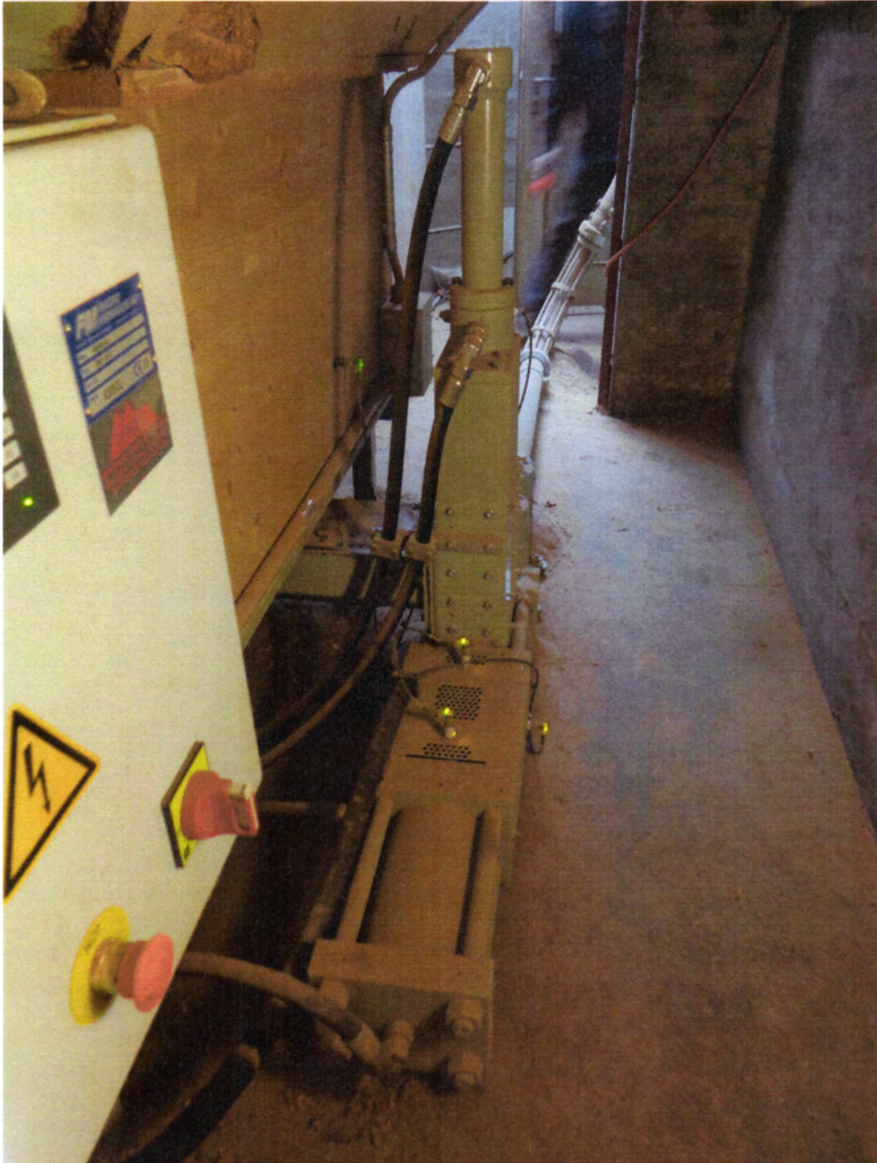
Ansicht Brikettieranlage mit Schaltkasten und Schubboden
